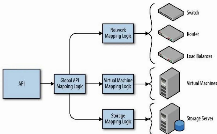
图 6-1: 将结构映射到资源的图表
