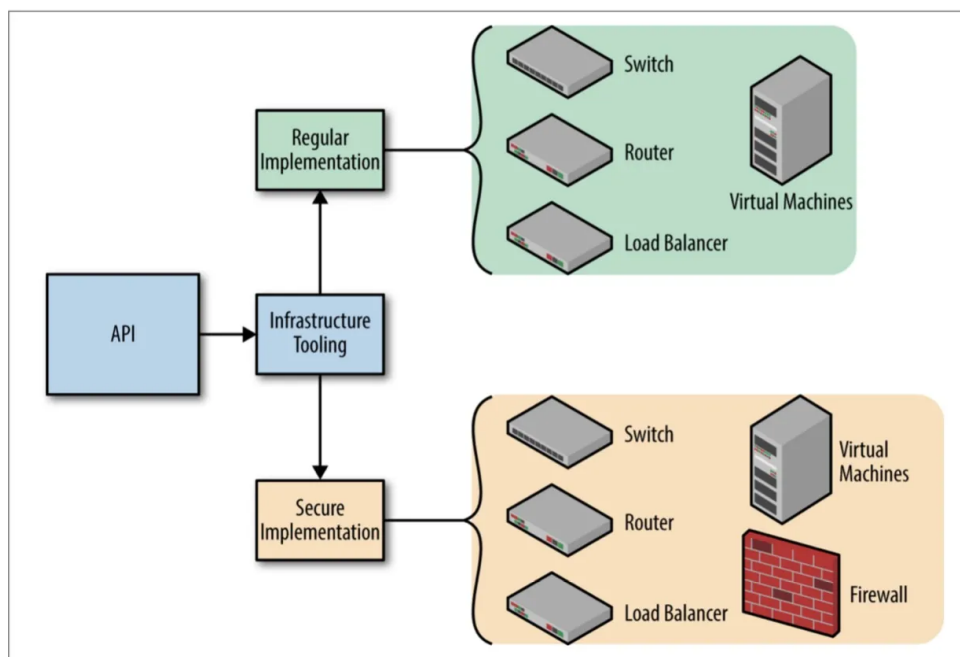
图 7-2: 一个 API 以不同的方式部署在同一个云中
