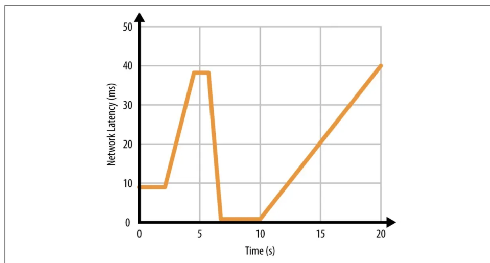
图 8-4: 包含网络故障的图形
