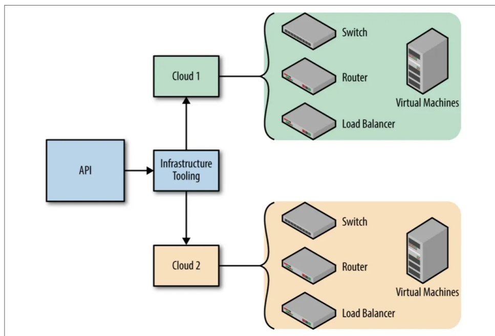
图 7-1: 一个 API 被部署在两个云中
