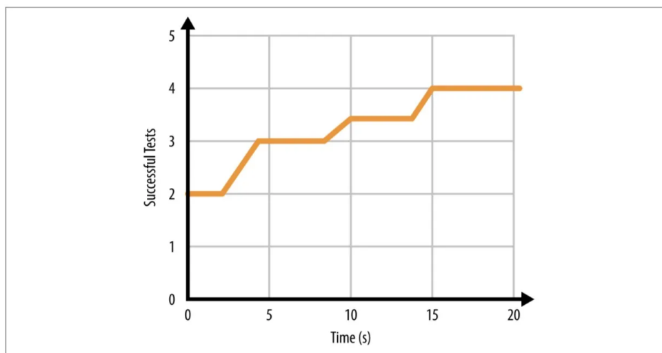
图 8-3: 成功的测试
